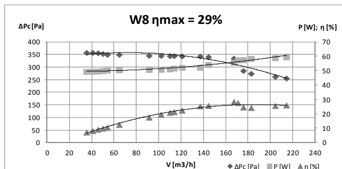
Fig. 9. Characteristics of fan W8
