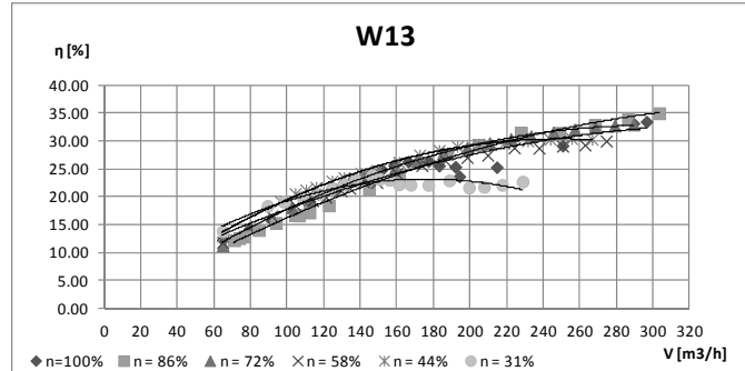
Fig. 16. Characteristics \eta for fan W13
