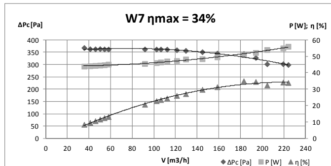
Fig. 8. Characteristics of fan W7
