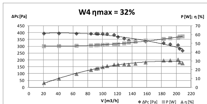
Fig. 5. Characteristics of fan W4
