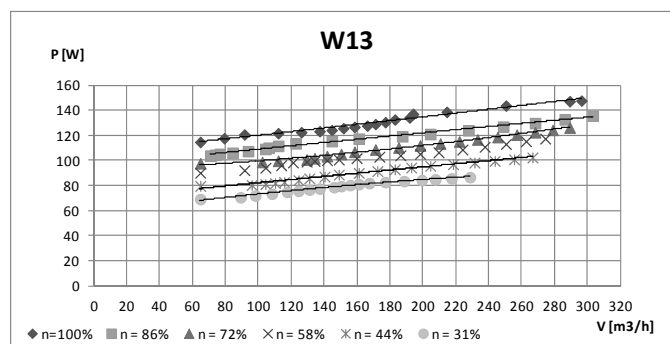
Fig. 15. Characteristics P for fan W13
